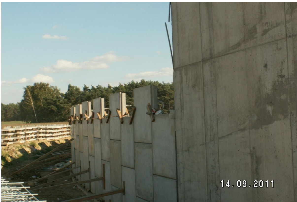
Ściana oporowa WD 213
